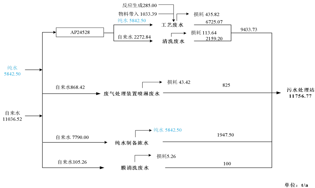
图 4.8-1 本项目水平衡图
