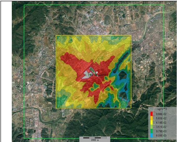
图 6.1.6-1 偏三甲苯叠加后日平均质量浓度分布图
