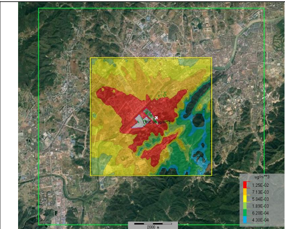
图 6.1.6-2 2,6-二氯苯酚叠加后日平均质量浓度分布图
