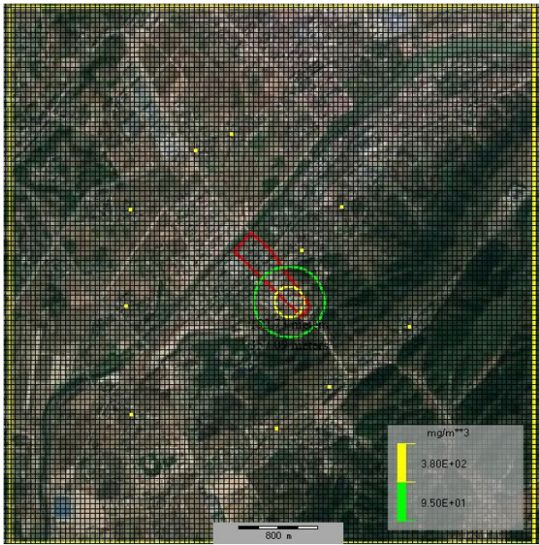
图 6.7.6-3 最不利气象条件下一氧化碳预测浓度达到不同毒性终点浓度的最大影响范围
