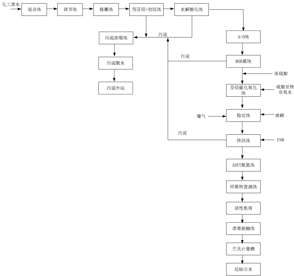
图 5.3.1-5 横店污水处理有限公司专业化工废水处理单元处理工艺流程图
