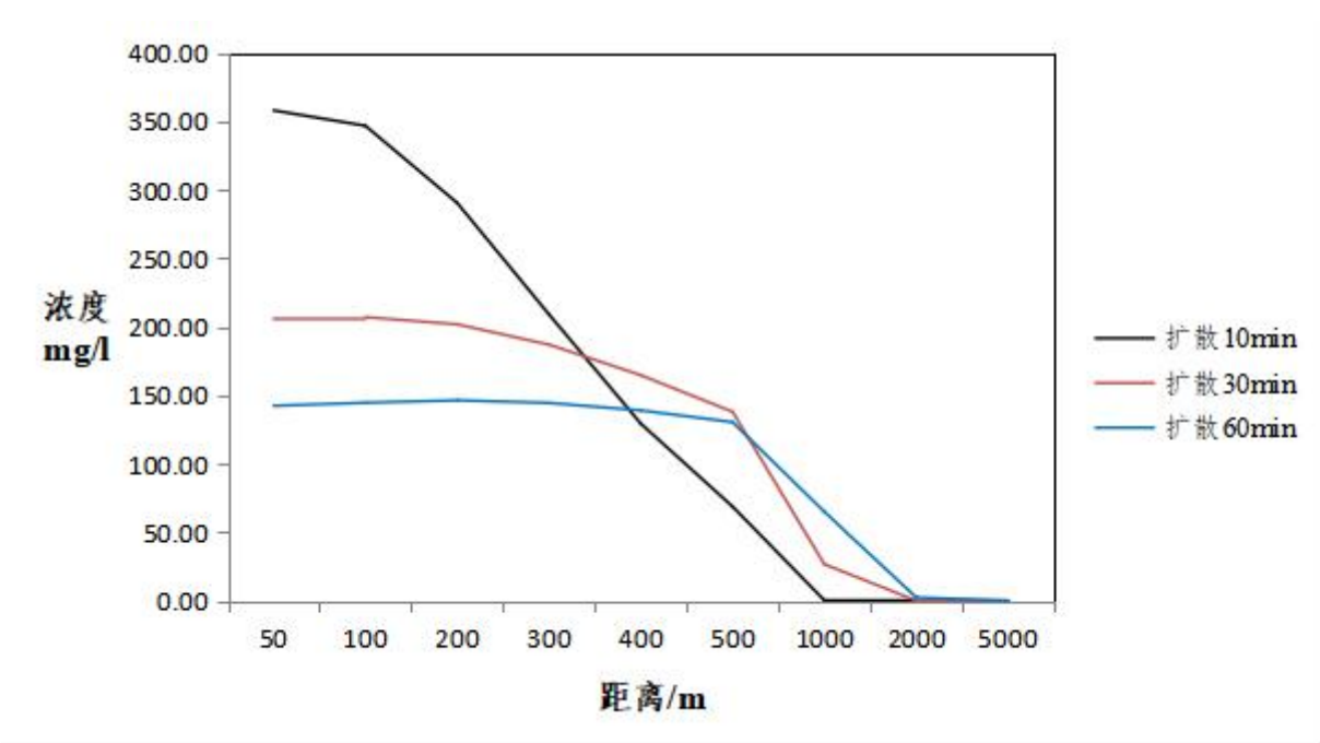
图 6.7.6.2-1 事故废水进入水体中 COD Cr 浓度扩散图 在 t 时刻，距离污染源下游 x=ut 处的污染物浓度峰值为：
