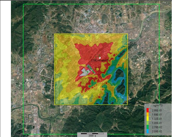
图 6.1.6-4 氯化氢叠加后日平均质量浓度分布图
