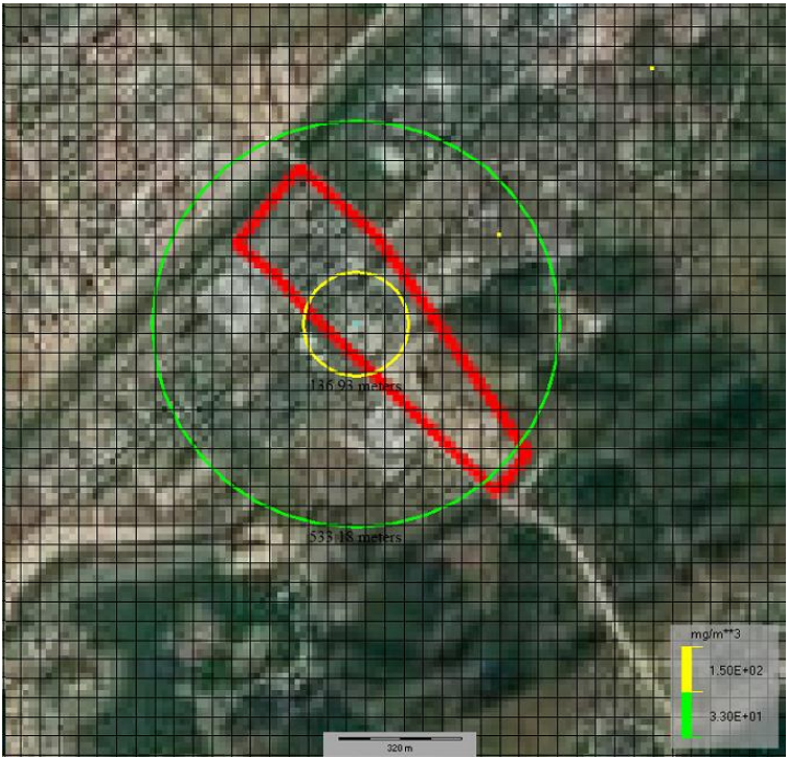
图 6.7.6-1 最不利气象条件下氯化氢预测浓度达到不同毒性终点浓度的最大影响范围
