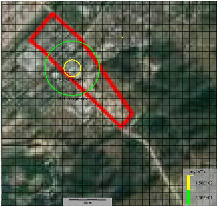
图 6.7.6-2 最常见气象条件下氯化氢预测浓度达到不同毒性终点浓度的最大影响范围
