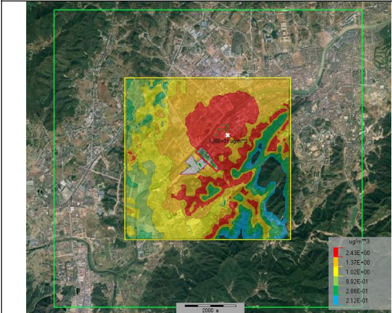
图 6.1.6-3 氯化氢叠加后小时平均质量浓度分布图
