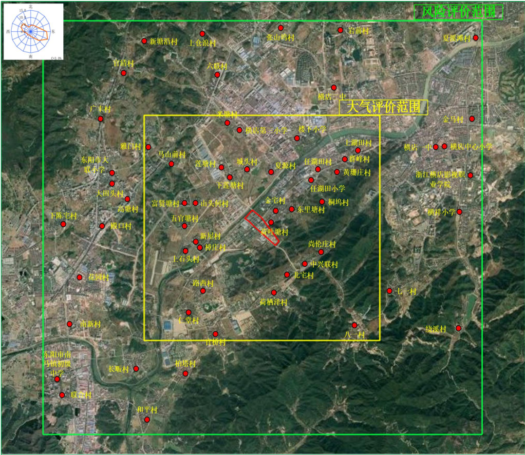
图 6.7.3-1 大气环境风险评价范围
