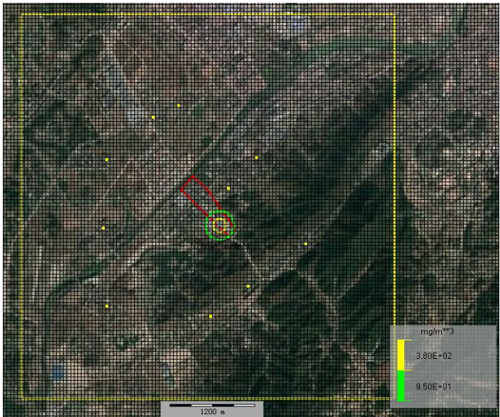
图 6.7.6-4 最常见气象条件下一氧化碳预测浓度达到不同毒性终点浓度的最大影响范围
