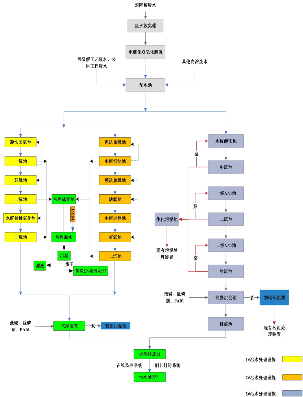
图 7.1.2-1 全厂污水处理站废水处理工艺流程图
